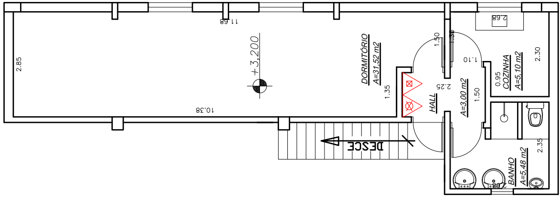
PLANTA PAVIMENTO SUPERIOR (ALOJAMENTO DOS FUNCIONÁRIOS) ESCALA: 1:50
