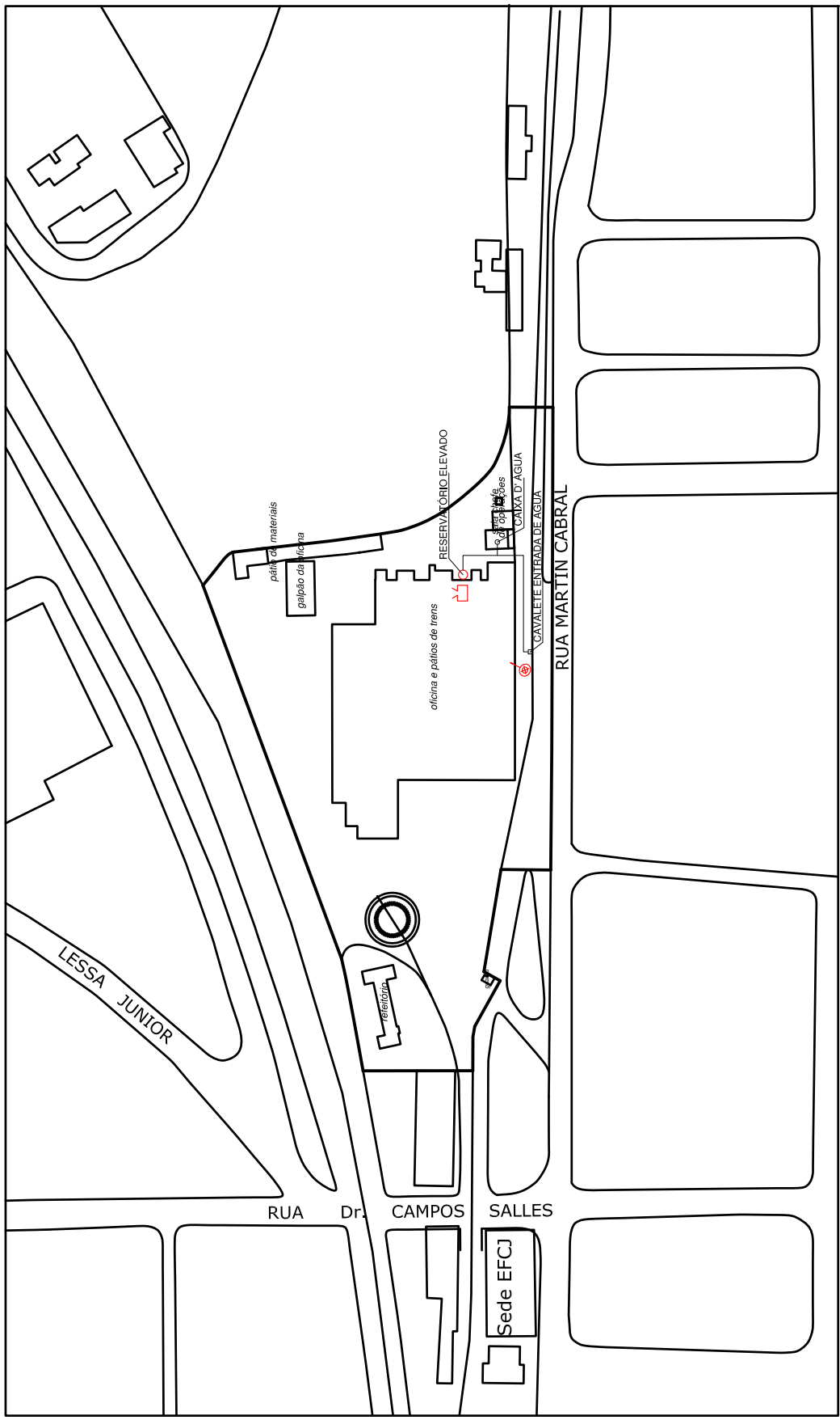
IMPLANTAÇÃO DE RISCO ESCALA: 1:2000
