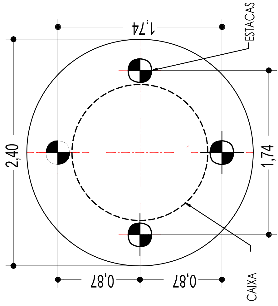
PLANTA DE FORMA ESC. 1:25
