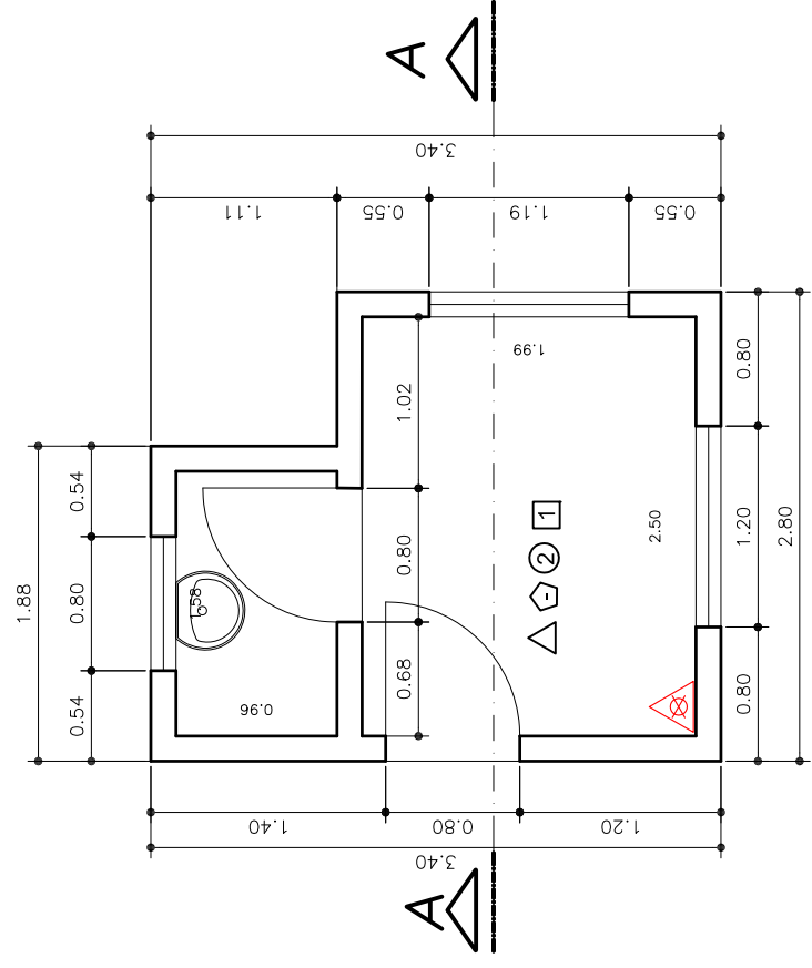
PLANTA GUARITA (PINDAMONHANGABA)
