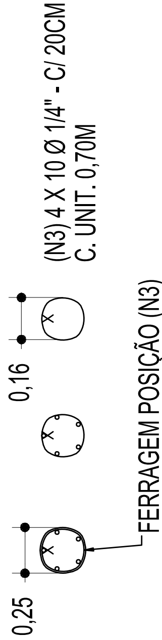
DETALHE DE ARMAÇÃO DAS ESTACAS ESC. 1:25
