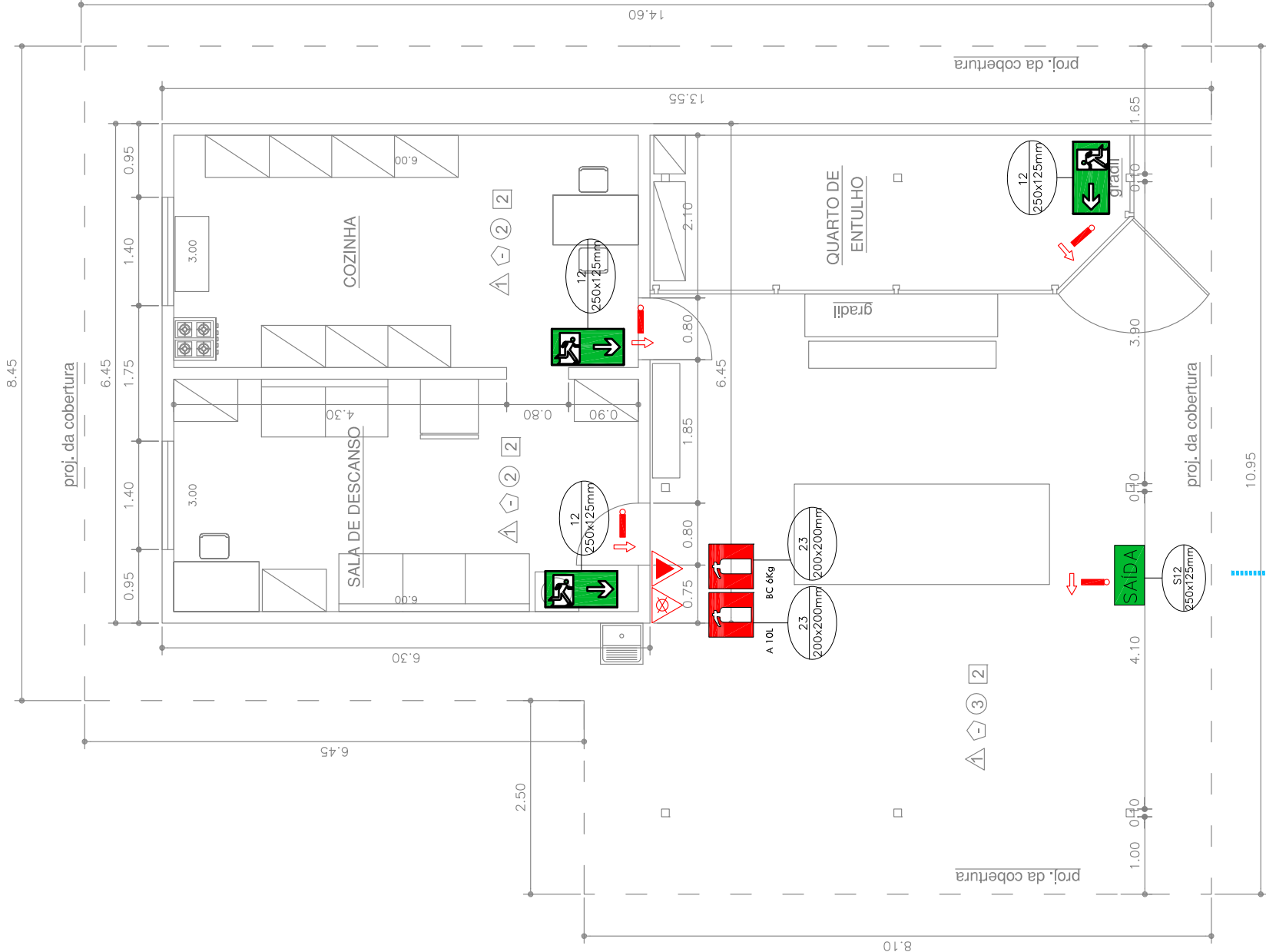
PLANTA BAIXA - SALA CHEFES DE OPERAÇÃO - INSTALAÇÕES E OBRAS
